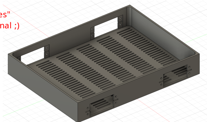
Figura 1: diseño del cuerpo.
