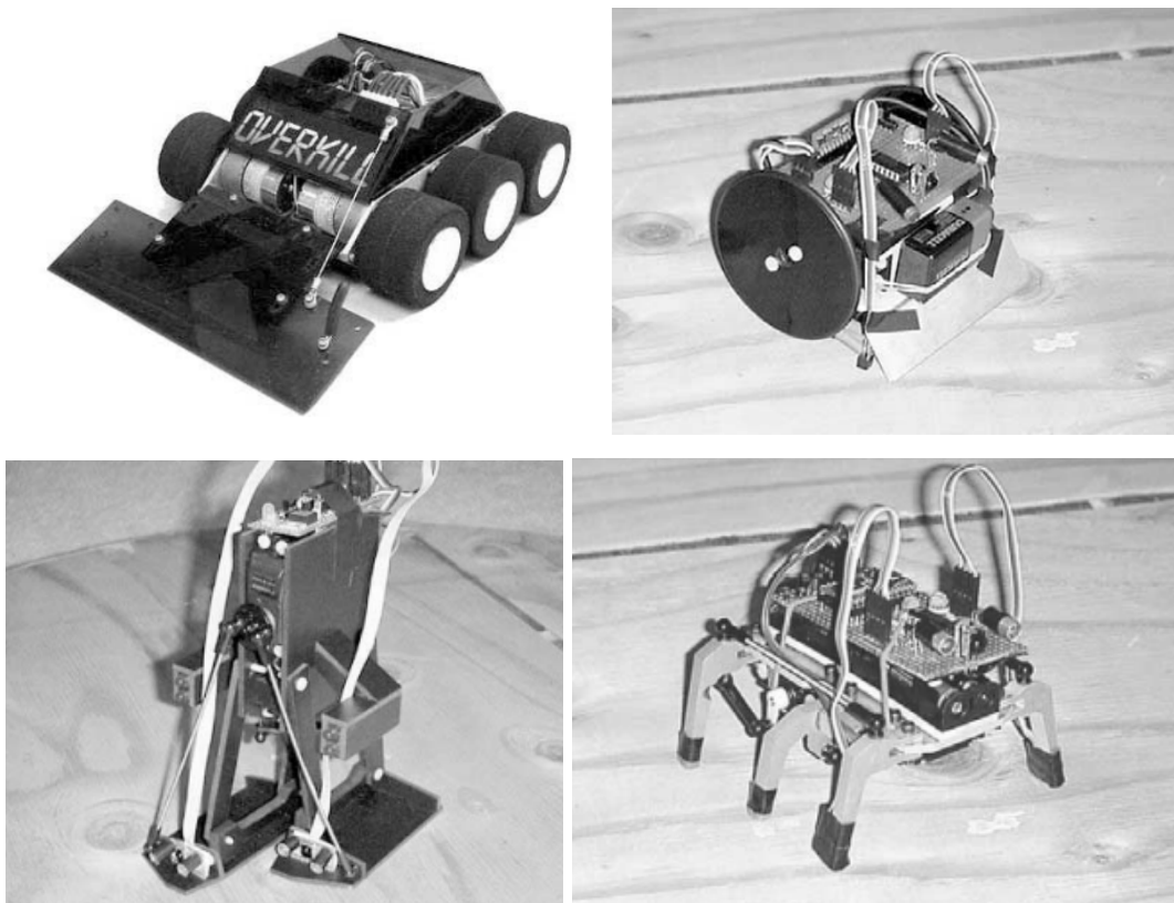
Fig. 6: Imagen del robot Overkill, Mini sumo, Biped Black Marauder y Hexapod Pete's Folly (de izquierda a derecha en orden descendente) (4)
