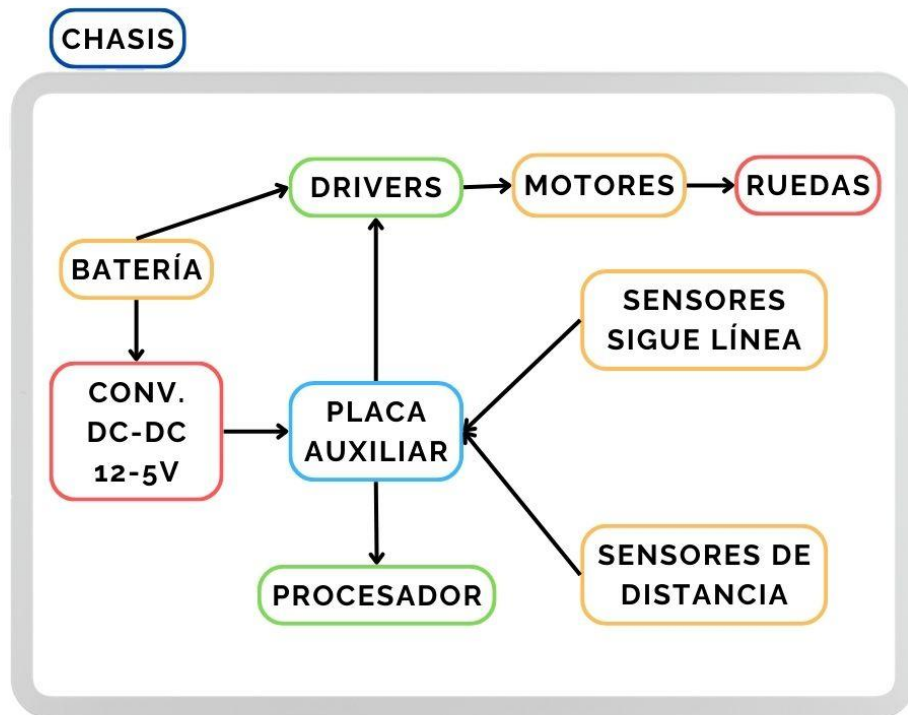
Fig. 9: Diagrama de subsistemas y conexiones
