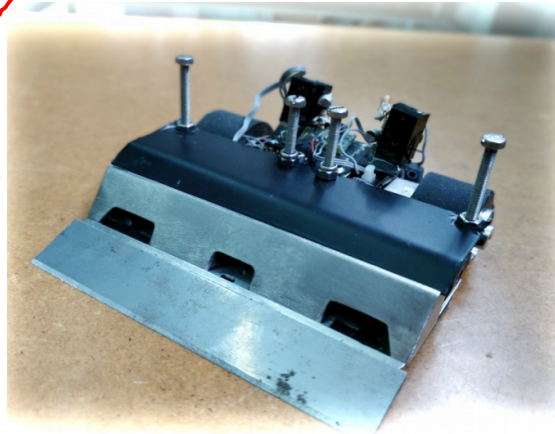
Fig. 7: Robot Smith Nightmare, 5 veces campeón de la LNRC.
