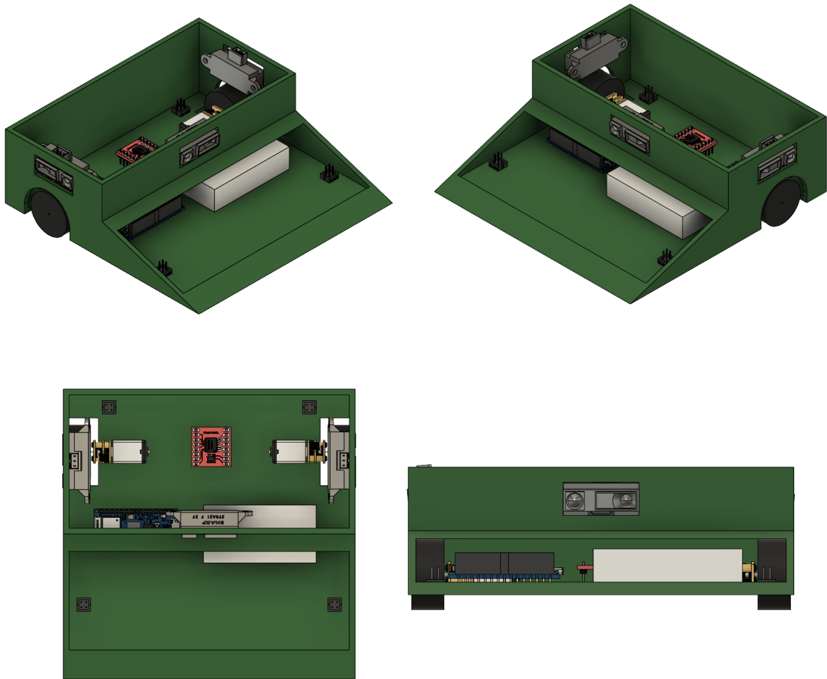
Fig. 20: Diferentes vistas del chasis con la posición de los componentes en su interior
